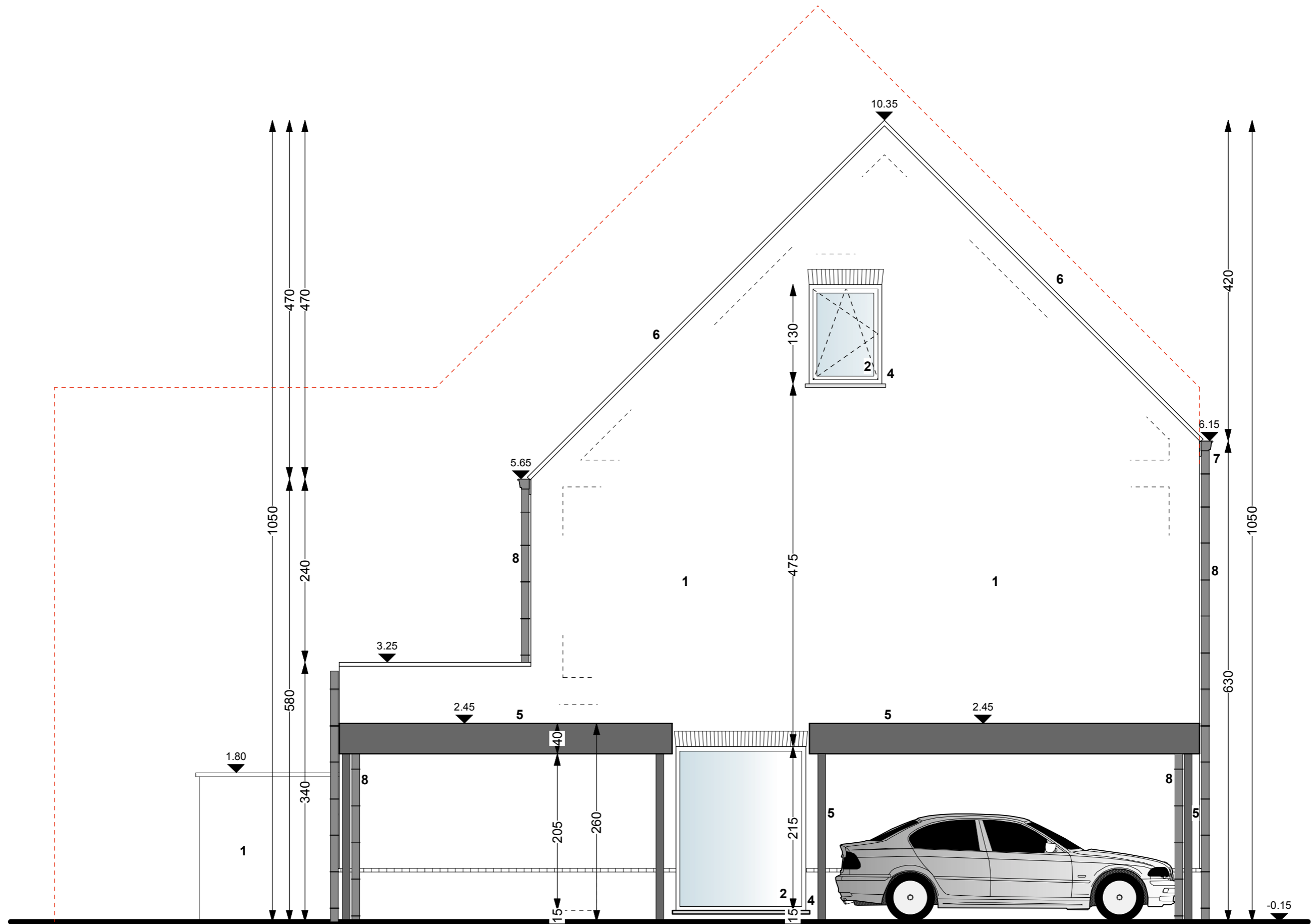
Linker zijgevel 1/50
