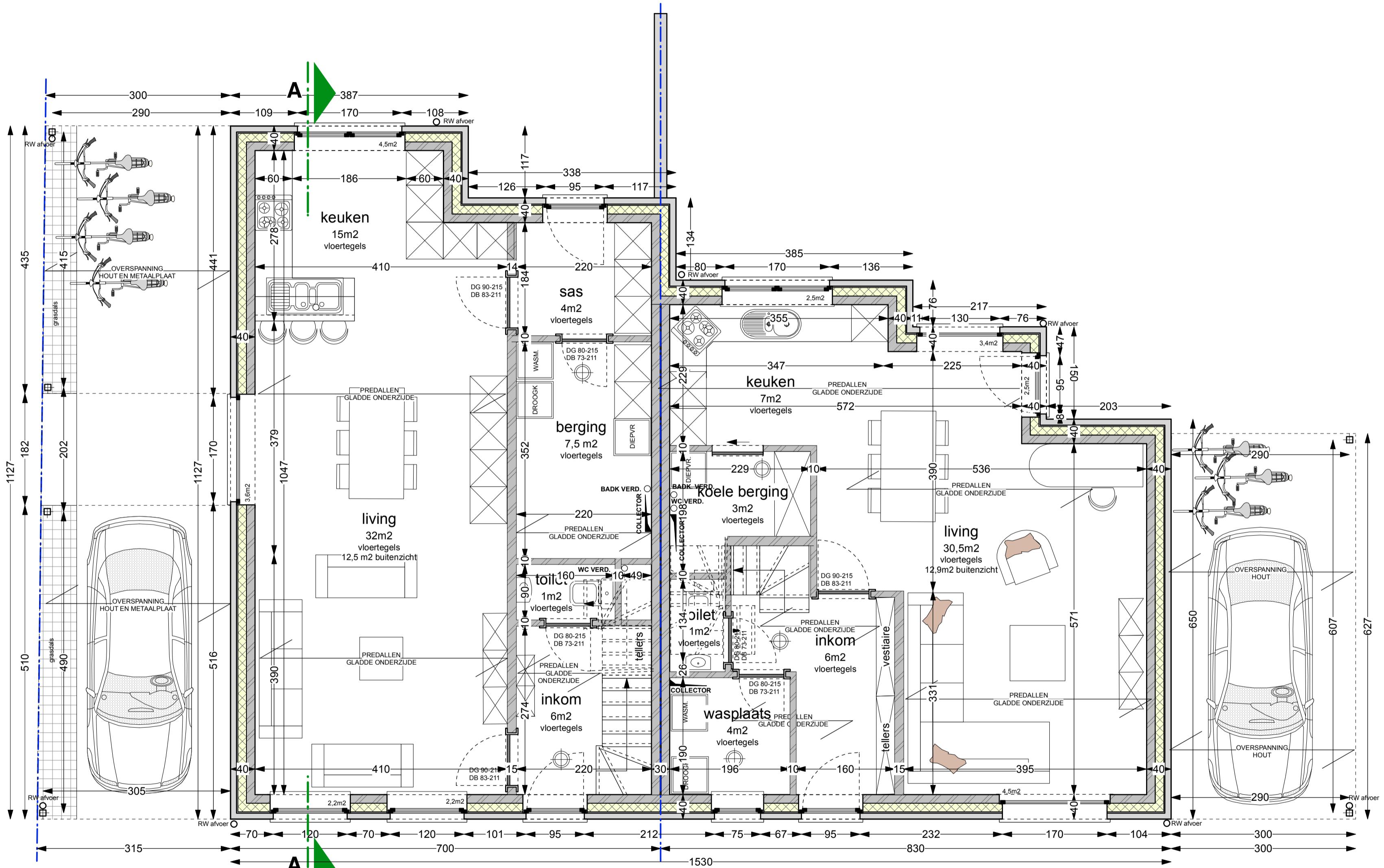
Grondplan 1/50 75 m 2 - 66 m 2
